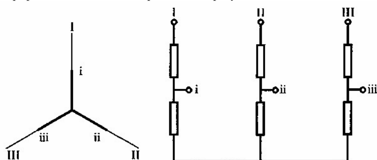
Рисунок Г.3 — Схема и группа соединения обмоток трехфазных автотрансформаторов (условное обозначение — V_{\text{авто}}=0 )
