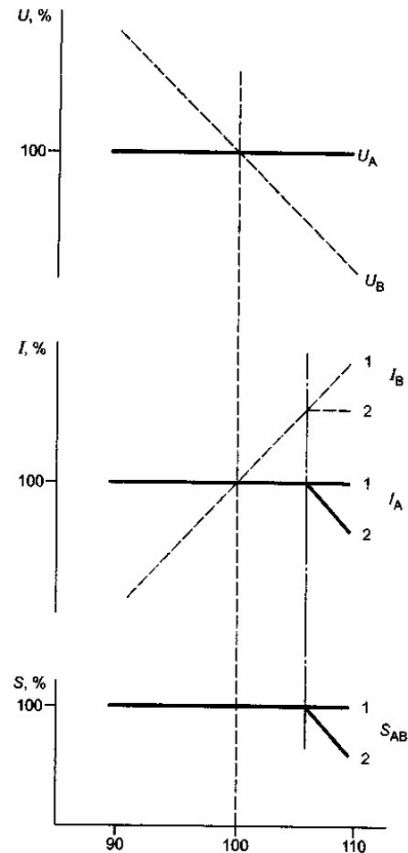
Коэффициент ответвления, %
