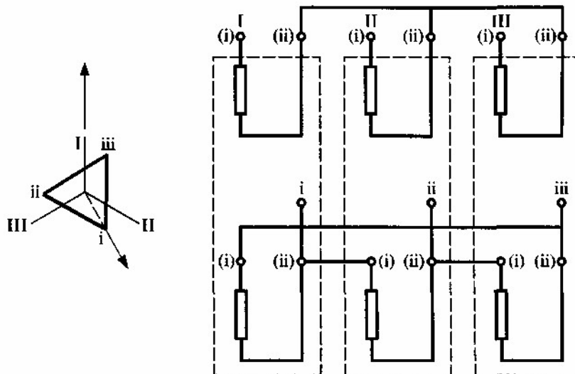
Рисунок Г.4 — Схема и группа соединения обмоток трехфазной группы однофазных трансформаторов (условное обозначение — У/Д—5)
