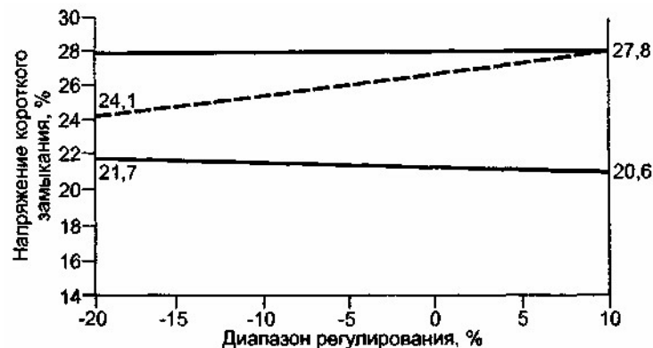
Рисунок В.1 — Диапазон изменения напряжения короткого замыкания
