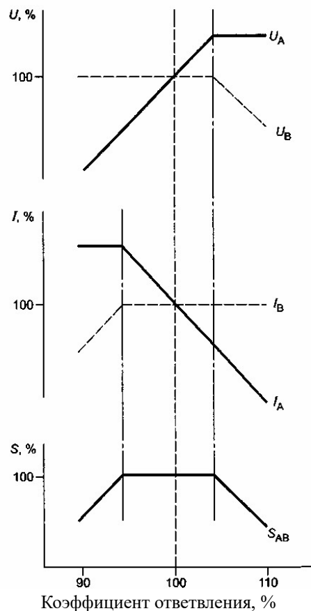
Рисунок 3 — Комбинированное регулирование напряжения (режим в)
