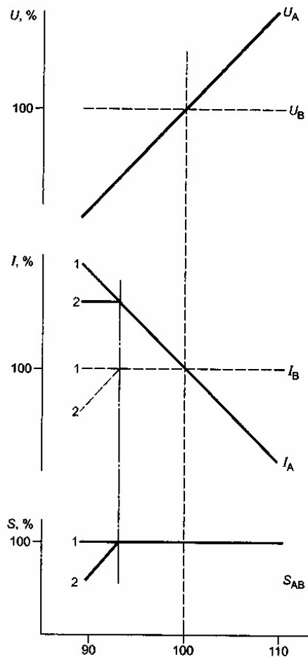
Коэффициент ответвления, %
